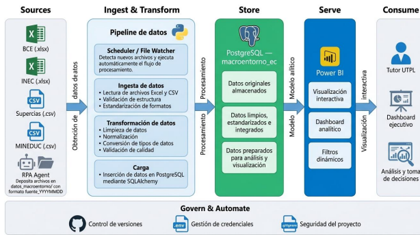
Figura 2. Arquitectura medallón del pipeline del Macroentorno Ecuador. Bronze almacena archivos crudos de RPA. Python transforma y carga en Silver (PostgreSQL). Las vistas Gold alimentan Power BI en tres paginas: P1 PIB, P2 empleo/VAB y P3 bachilleres-empresas.
